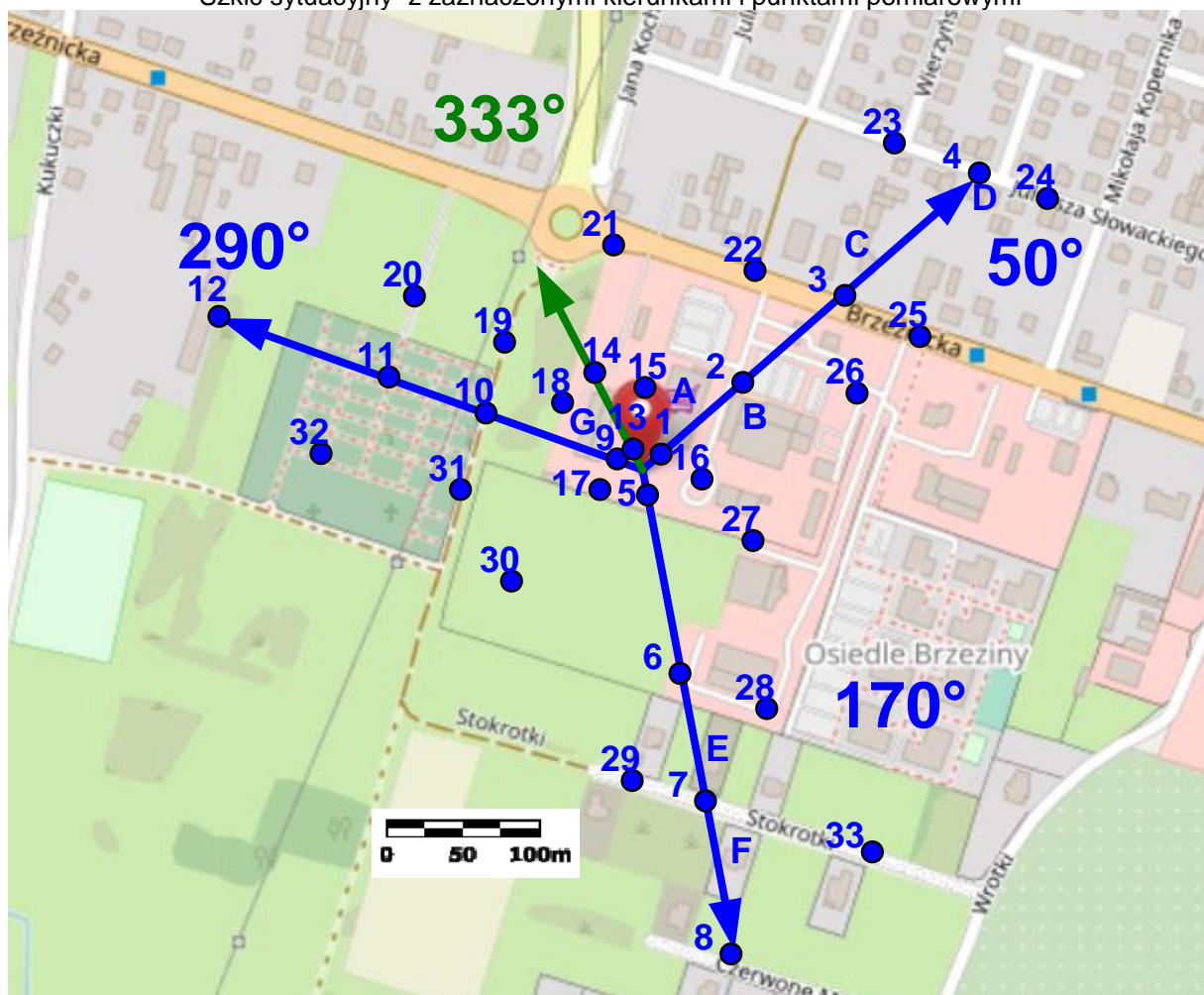
Szkiec sytuacyjny z zaznaczonymi kierunkami i punktami pomiarowymi
