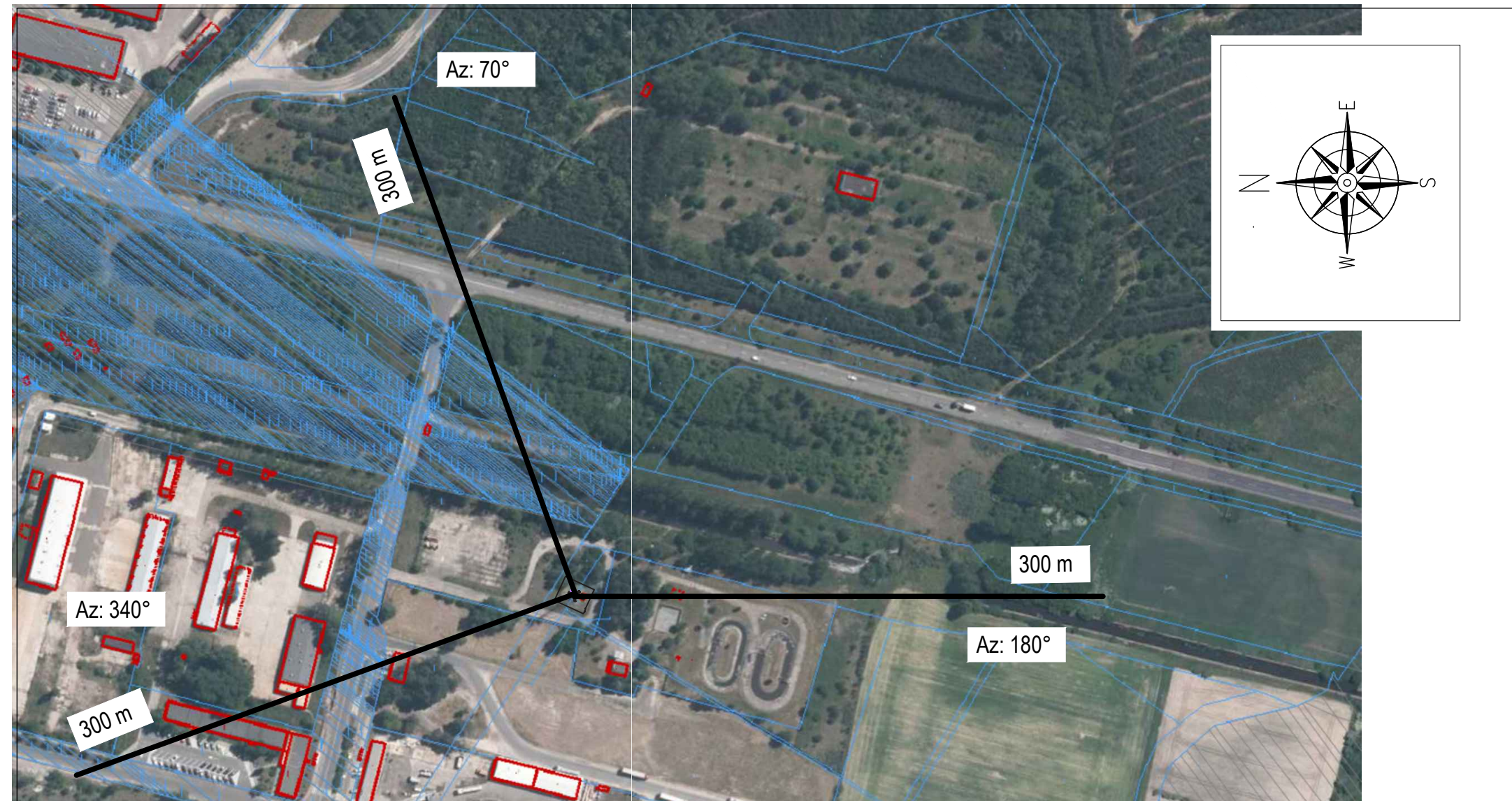
Rys. 1. Rzut poziomy osi głównej wiązki promieniowania w odległości do 70 i 300 metrów od środka elektrycznego anten sektorowych.
